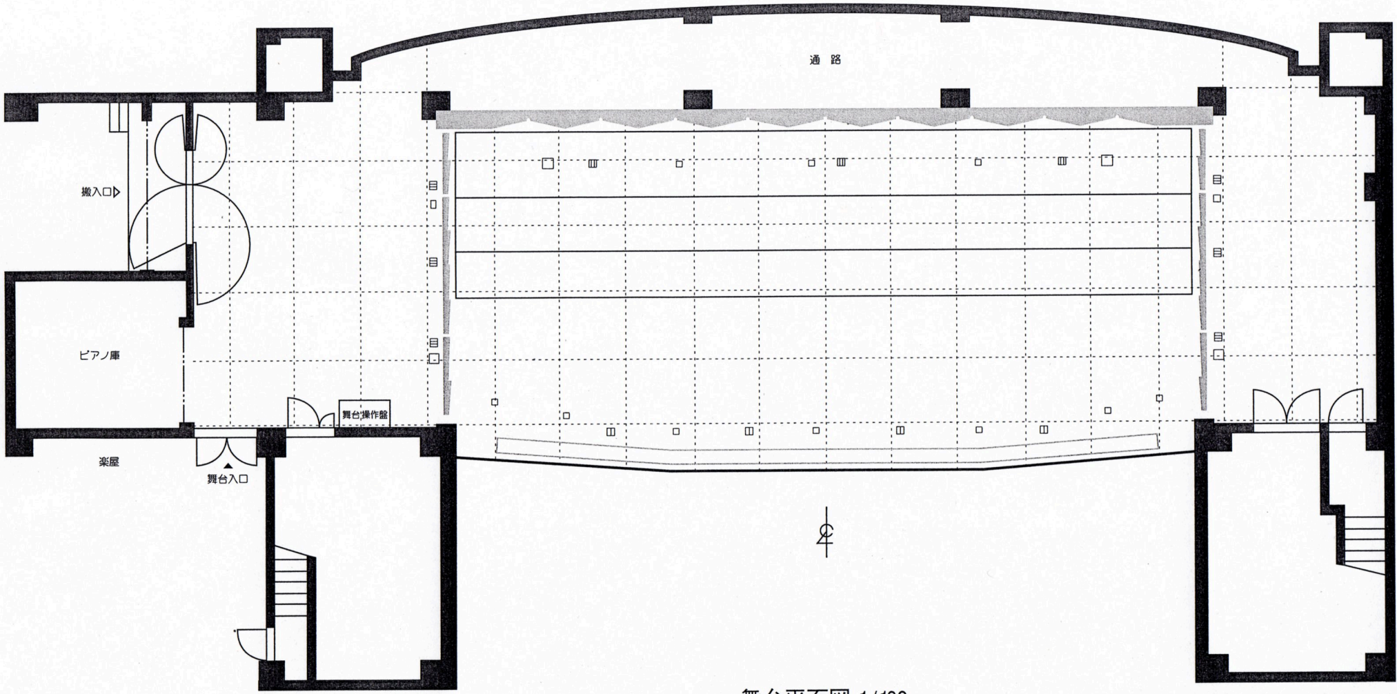
舞台平面図 1/100
